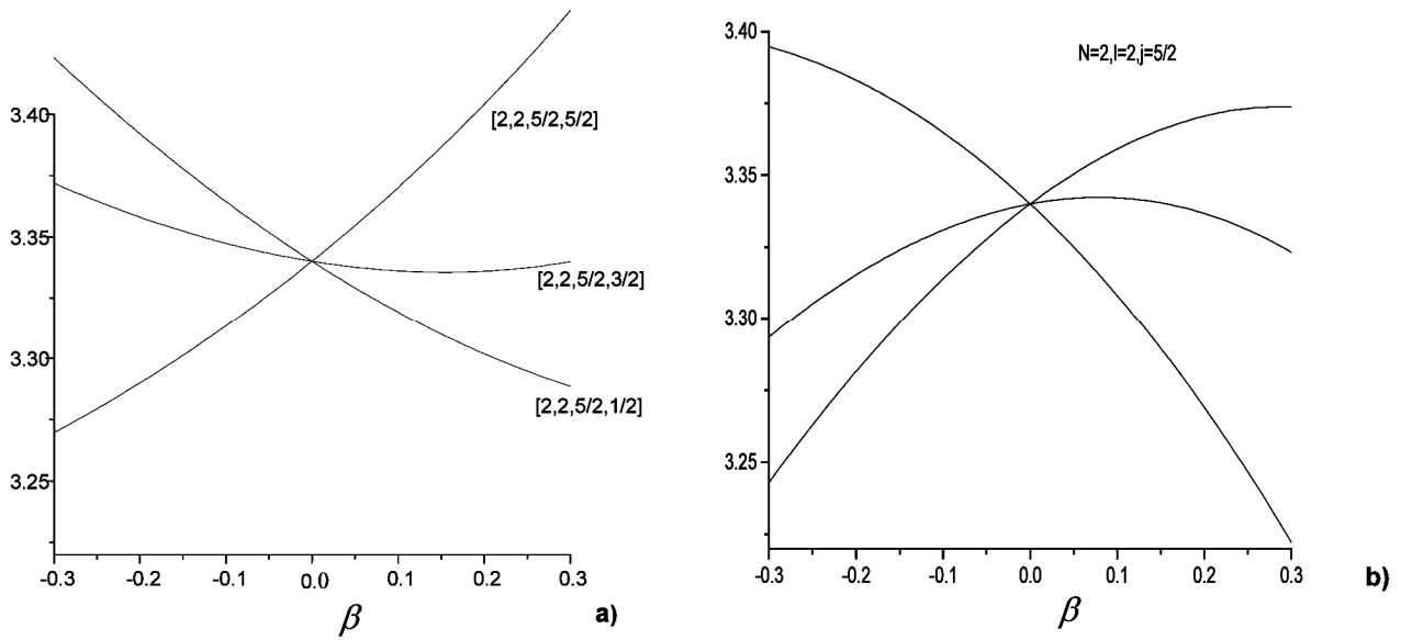
شکل ۴. ترازهای مختلف انرژی به واحد \hbar\omega برحسب پارامتر تغییر شکل \beta (a: مدل نیلسون N=2 و l=2 ، j=\frac{5}{4} و (b) مدل تغییر شکل یافته سه محوری N=2 و l=2 ، j=\frac{5}{4} ).
