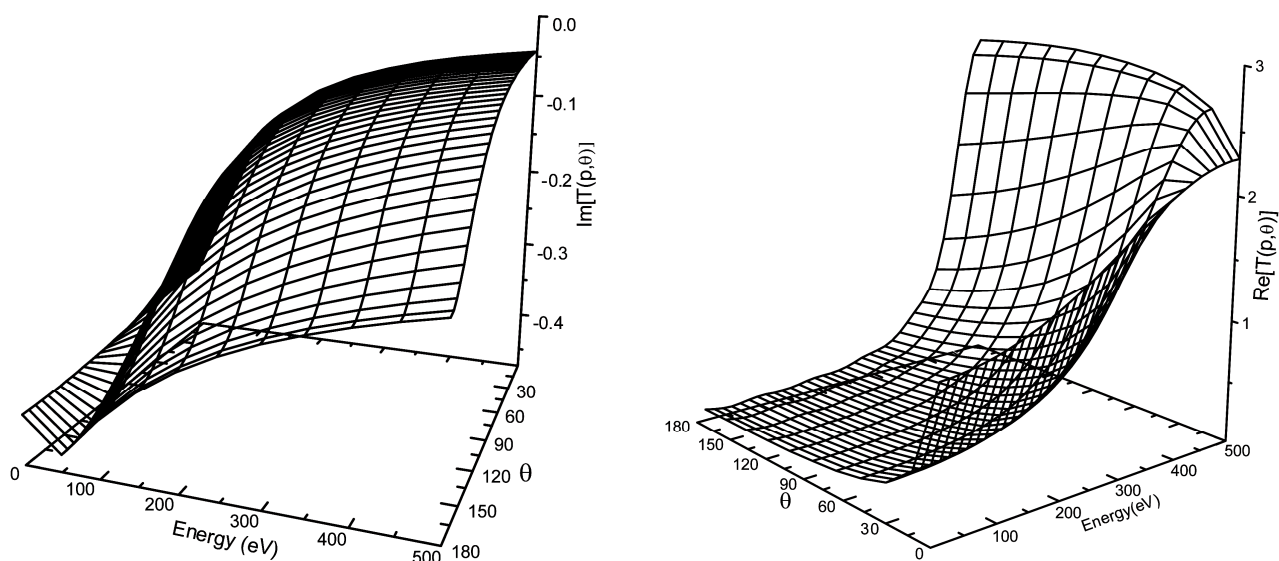
شکل ۳. مقادیر حقیقی و موهومی ماتریس گذار بر روی پوسته انرژی به ازای گستره انرژی ۵۰۰-۱۰ eV و زوایای پراکندگی ۱۸۰-۰ درجه.
