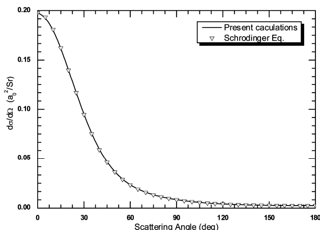
شکل ۷. مقایسه نتایج به دست آمده، با استفاده از روش حاضر، با نتایج حاصل از معادله شرودینگر برای توزیع زاویه‌ای سطح مقطع جزیی پراکندگی به ازای انرژی فرودی ۱۰۰ eV و زوایای پراکندگی ۰-۱۸۰ درجه.
