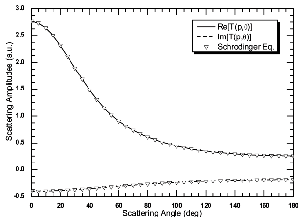
شکل ۶. مقایسه نتایج به دست آمده، با استفاده از روش حاضر، با نتایج حاصل از معادله شرودینگر برای مقادیر حقیقی و موهومی ماتریس گذار بر روی پوسته انرژی به ازای انرژی ۱۰۰ eV و زوایای پراکندگی ۰-۱۸۰ درجه.
