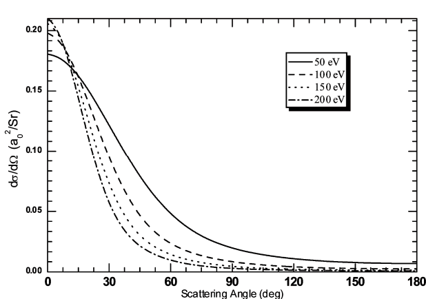
شکل ۵. توزیع زاویه‌ای سطح مقطعهای جزئی پراکندگی به ازای انرژیهای فرود ۵۰، ۱۰۰، ۱۵۰ و ۲۰۰ eV.
