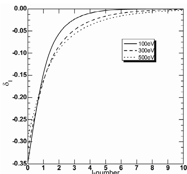
شکل ۲. تغییرات جابجایی فاز: الف) بر حسب انرژی پراکندگی به ازای اعداد کوانتومی مداری ۵- و ۰ (ب) بر حسب عدد کوانتومی مداری به ازای انرژیهای فرودی ۱۰۰، ۳۰۰ و ۵۰۰ eV.
