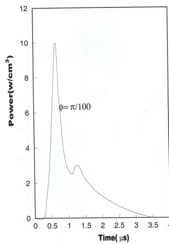
شکل ۲. در این شکل توان خروجی لیزر برای تزریق خارجی \Delta Wk/cm^2 و \phi = \pi/100 رسم شده است.
