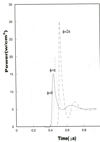
شکل ۱. در این شکل توان خروجی لیزر برای تزریق خارجی \Delta W/cm^2 در سه حالت \phi = 0 ، \phi = \pi و \phi = 2\pi به ترتیب منحنیهای پیوسته، نقطه چین و خط چین با هم مقایسه شده است.
