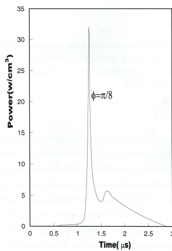
شکل ۳. در این شکل توان خروجی لیزر برای تزریق خارجی \Delta Wk/cm^2 و \varphi = \pi/8 رسم شده است.
