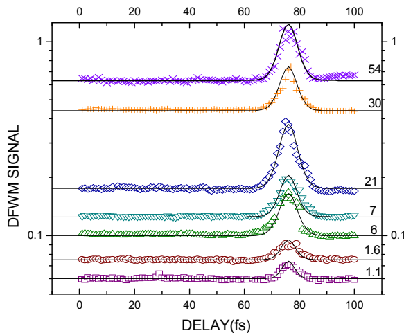
شکل ۸. سیگنالهای ترکیب چهار موج تبهگن بر حسب تاخیر زمانی پرتو کاوشگر در لایه چلکا جنید نشان داده شده اند. اعداد نشان داده شده در بالای هر نمودار نشان دهنده شدت پرتو ورودی بر حسب \text{GW/cm}^2 می باشند.
