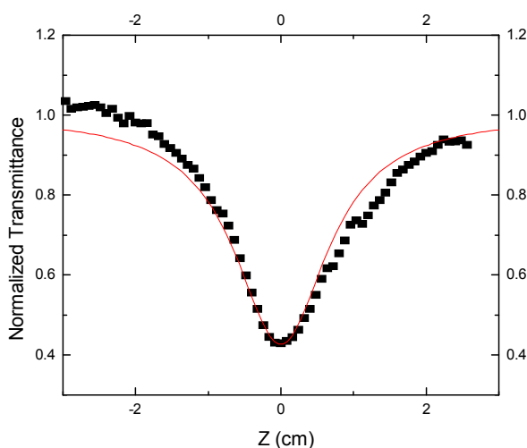
شکل ۱۱. نمودار برازش منحنی نظریه تراگسیلندگی با نتایج تجربی برای ماده S_p S_p AS_p . مقدار ضریب جذب دو فوتونی \beta = 0.29 \frac{cm}{GW} محاسبه شده است.
