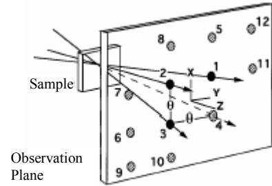
شکل ۳. آزمایش ترکیب چهار موج تبهگن در حالت روش جلویی (forward). پرتوهای ۱ و ۲ و ۳ تقریباً در جهت z منتشر می‌شوند.
