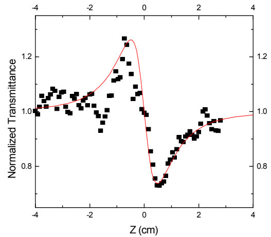
شکل ۱۲. نمودار برآزش منحنی نظریه تراگسیلندگی حالت شکاف بسته با نتایج تجربی برای ماده چلکا جنید. مقدار ضریب شکست غیرخطی برابر با \frac{m^2}{W} \times 10^{-17} \times 3 می‌باشد.
