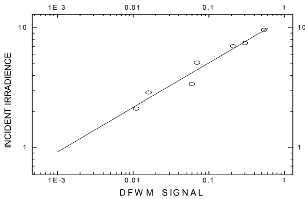
شکل ۱۳. سیگنال ترکیب چهار موج تبهگن بر حسب شدت پرتو ورودی در ماده چلکا جنید نشان داده شده است. برآزش داده‌ها وابستگی به شدت را به صورت I^{2/57 \pm 0/25} نشان می‌دهد. واحدها اختیاری هستند.
