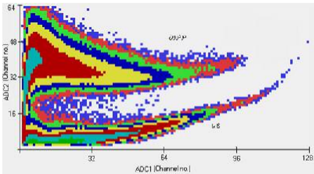
شکل ۵. طیف جداسازی شده نوترون و گاما در برهم‌کنش D+^4Be با دوترون‌های ۱۰ MeV در زاویه ۱۰ درجه.
