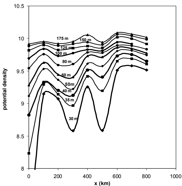
شکل ۵. ج) نمودار تغییرات افقی چگالی پتانسیل ( \text{kg/m}^3 ) برحسب فاصله از ساحل جنوبی دریای خزر در امتداد محور جنوبی - شمالی در اعماق مختلف (به طوری که به ترتیب ۳۰ و ۳۵ و ۴۰ و ۵۰ و ۶۰ و ۸۰ و ۱۰۰ و ۱۲۵ و ۱۵۰ و ۱۷۵ متر می‌باشند).
