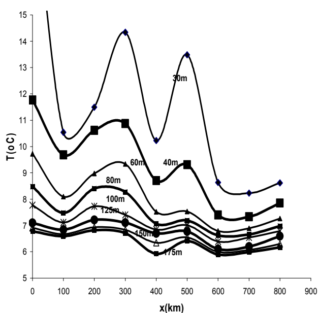
شکل ۵. الف) نمودار تغییرات افقی دما برحسب فاصله از ساحل جنوبی دریای خزر در امتداد محور جنوبی - شمالی در اعماق مختلف (به طوری که به ترتیب ۳۰ و ۴۰ و ۶۰ و ۸۰ و ۱۰۰ و ۱۲۵ و ۱۵۰ و ۱۷۵ متر می‌باشند).
