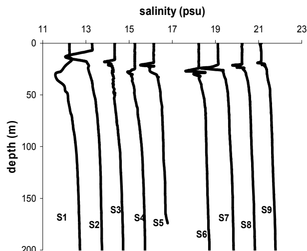
شکل ۴. نیمرخهای قائم شوری برای ایستگاههای مختلف از ۱ تا ۹ (برای بررسی واضحتر به اندازه‌های ایستگاه ۲ یک واحد، ایستگاه ۳ دو واحد و ..... اضافه شده است).
