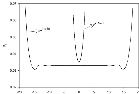
شکل ۵. چگالی مایع با مولکولهای بیضی‌وار بر حسب فاصله کاهش یافته برای 0.276 \eta و حالتی که فاصله بین دو دیوار 8a و 40a باشند.
