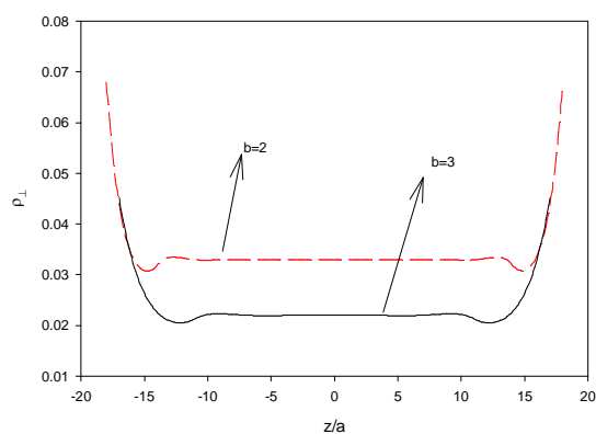
شکل ۶. چگالی مایع با مولکولهای بیضی‌وار عمود بر دیواره‌ها بر حسب فاصله برای 0.276 \eta و 3 و 2 b/a .
