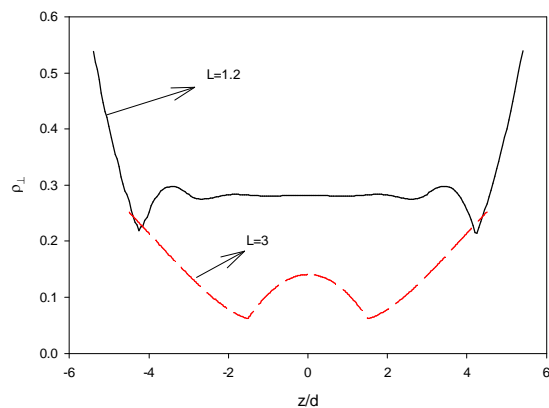
شکل ۲. چگالی بلور مایع با مولکولهای استوانه‌ای دوار بر حسب فاصله کاهش یافته تا دیواره‌ها برای حالتی که کسر به هم پکیدگی \eta = 0.265 و l = 1/2 و 3 می‌باشد.
