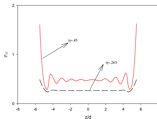
شکل ۳. چگالی بلور مایع با مولکولهای استوانه‌ای دوار بر حسب فاصله کاهش یافته از دو دیواره‌ها برای l/d = 1/2 و کسر به هم پکیدگی 0.265 و 0.45 \eta .
