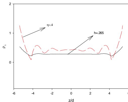
شکل ۱. چگالی بلور مایع با مولکولهای استوانه‌ای دوار بر حسب فاصله کاهش یافته تا دیواره‌ها برای l/d = 1/2 و دو حالت 0.4 و 0.265 \eta .
