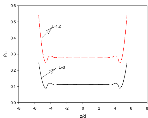
شکل ۴. چگالی بلور مایع با مولکولهای استوانه‌ای دوار بر حسب فاصله کاهش یافته از دو دیوار برای کسر به هم پکیدگی \eta = 0.265 و 3 و l/d = 1/2 .
