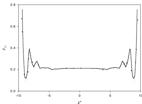
شکل ۸ چگالی بلور مایع با مولکولهای بیضی وار موازی دیوارهها برحسب فاصله کاهش یافته، برای کسر پکیدگی 0/5 و نسبت قطر بزرگ به قطر کوچک 5 خط ممتد مربوط به محاسبت این مقاله و نقاط مربوط به نتایج شبیهسازی مونت-کارلو می باشند.
