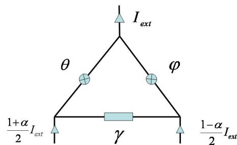
شکل ۲. آرایه مثلثی مورد مطالعه، پیوندگاههای q و j توسط پیوندگاه g با هم جفت شده‌اند. a میزان از عدم تقارن در توزیع جریان است.
