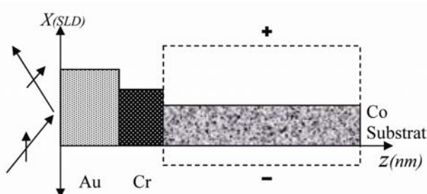
شکل ۱. نمونه دو لایه‌ای طلا - کروم بر روی زیر لایه مغناطیسی کبالت - نقاط خط چین SLD موثری است که توسط نوترون‌های قطبیده در جهت موازی و پاد موازی میدان مغناطیسی حاصل از مغناطش زیر لایه، تجربه می‌شود.
