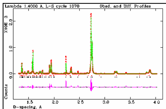
شکل ۱. نمایه پراش در دمای اتاق در حالتی که 0.6 < x < 0.7 می‌باشد.
