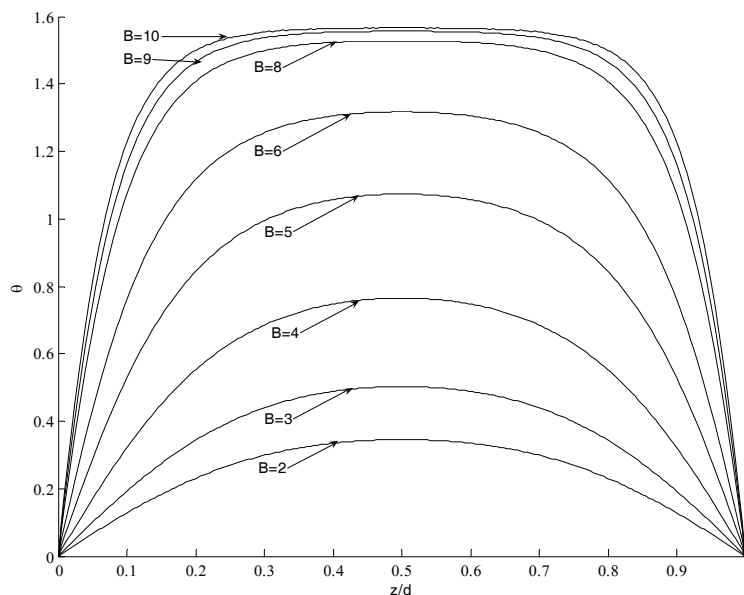
شکل ۱. توزیع میدان جهت نما در شرایط چنگ زدگی نامتناهی، تغییرات امتداد جهت نما بر حسب ضخامت بدون بعد Z/d ، به ازای میدان های مغناطیسی متغیر به ترتیب از B=10T تا B=1T .
