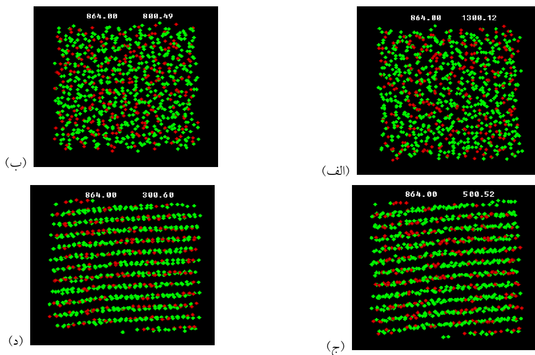
شکل ۶. ساختارهای بلوری آلیاژ Ag-۸%Au در دماهای مختلف، الف) ۱۳۰۰ K، ب) ۸۰۰ K، ج) ۵۰۰ K، د) ۳۰۰ K.
