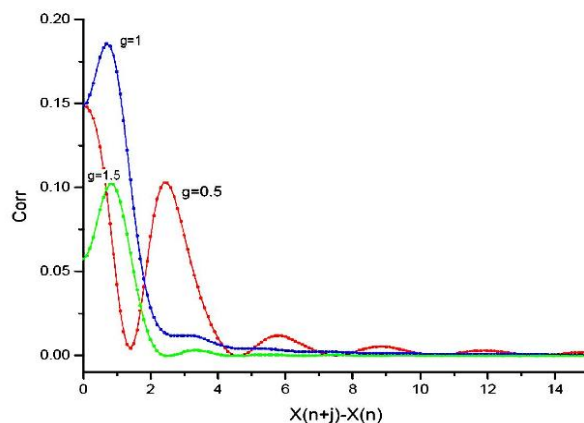
شکل ۵. نمودار تابع همبستگی C^x(j) برحسب فاصله، به ازای سه مقدار متفاوت g = 0.5, 1, 1.5 . همان طور که مشاهده می‌شود، با افزایش فاصله، همبستگی اسپینی کاهش می‌یابد.
