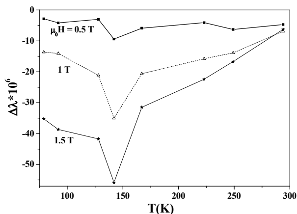
شکل ۱۱. وابستگی دمایی منحنی‌های مغناطوتنگش ناهمسانگرد \text{Nd}_6\text{Fe}_{13}\text{Cu} ( \Delta\lambda ) نمونه ۱۱.
