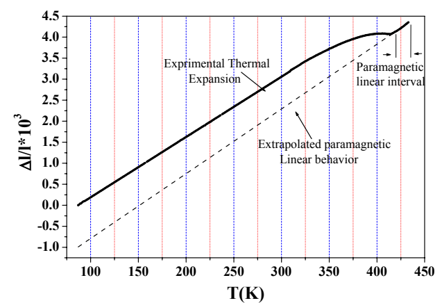
شکل ۸. منحنی انبساط گرمایی تجربی نمونه \text{Nd}_6\text{Fe}_{13}\text{Cu} در گستره دمایی 80 تا 450 کلوین. خط چین، برون‌یابی رفتار پارامغناطیسی به کمتر از دمای نیل ( T_N = 419 \text{ K} ) را نشان می‌دهد.
