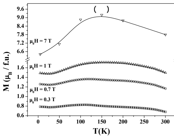
شکل ۶. تغییرات مغناطش بر حسب دما در چند میدان مغناطیسی انتخابی برای نمونه‌های Nd_7Fe_{13-x}Co_xCu (الف) x = 0 و (ب) x = 1 .
