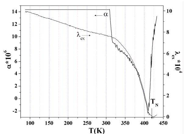
شکل ۹. وابستگی دمایی مغناطوتنگش خودبه‌خودی و ضریب انبساط گرمایی نمونه \text{Nd}_6\text{Fe}_{13}\text{Cu} .
