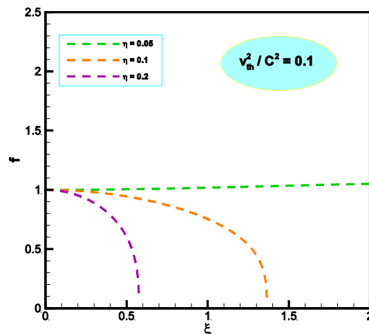
شکل ۱۱. تغییر پهنای لیزر با فرض \eta = 0.08, 0.1, 0.2 و v_{th}^2 / C^2 = 0.1 .
