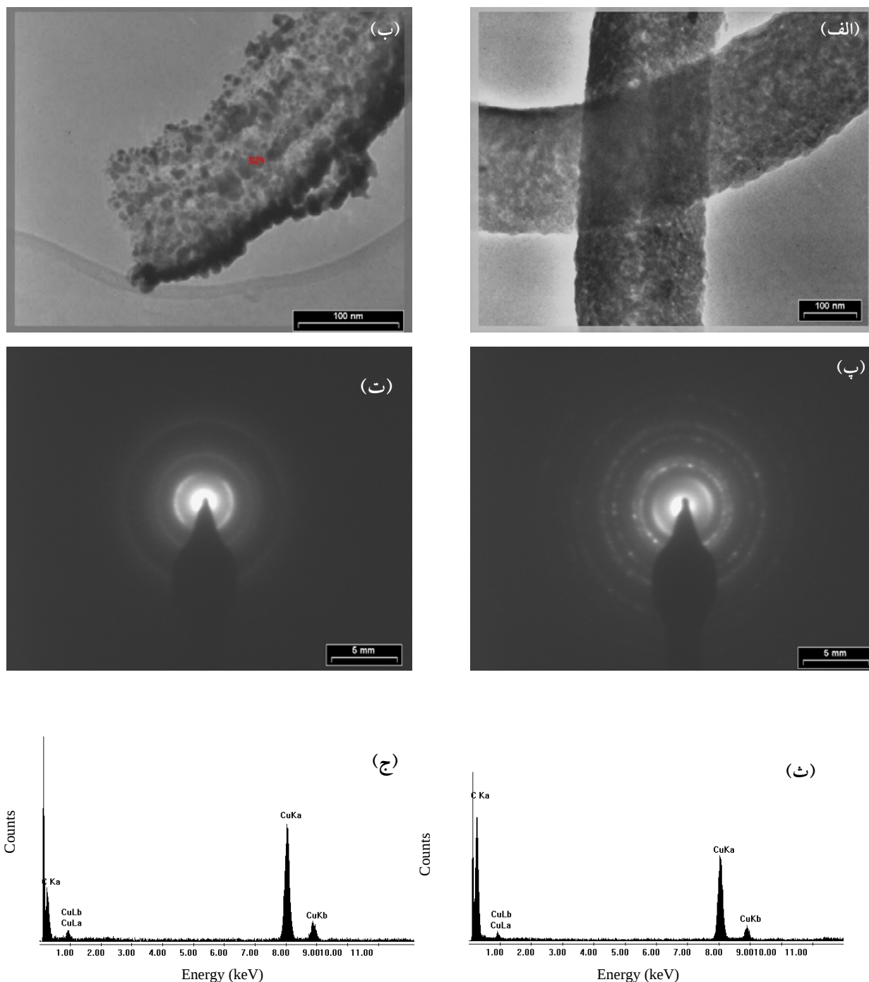
شکل ۳. تصاویر TEM نانو فیبرهای کربنی رشد یافته در دمای 800^{\circ}\text{C} بر روی نانو ذرات کاتالیستی نیکل لایه نشانی شده برای زمان‌های ۱ و ۳ دقیقه به ترتیب در (الف) و (ب). الگوهای پراش (SAED) آنها به ترتیب در (پ) و (ت) و طیف‌های EDX آنها به ترتیب در (ث) و (ج) نشان داده شده‌اند.
