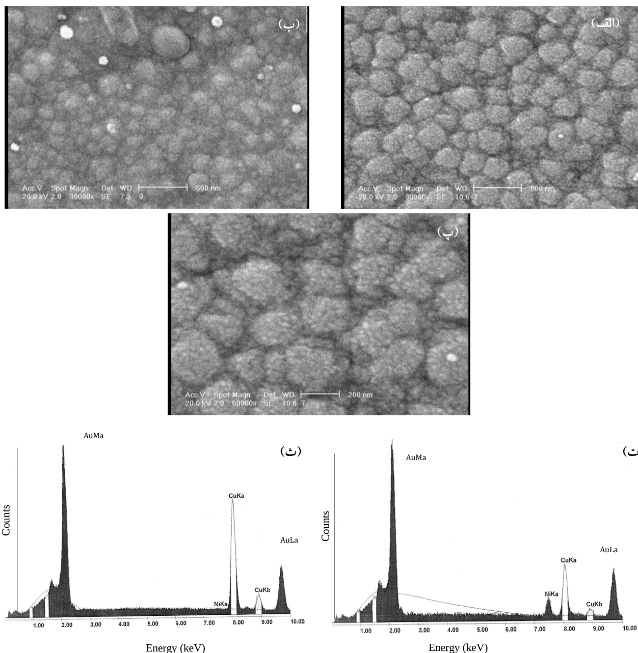
شکل ۱. تصاویرهای SEM لایه‌های کاتالیستی نیکل انباشته در دمای 350^{\circ}\text{C} برای زمان‌های الف و پ) ۳ و ب) ۱ دقیقه، طیف‌های EDX زیرلایه مسی و لایه کاتالیستی نیکلی انباشته بر روی آن به ترتیب در (ت) و (ث).
