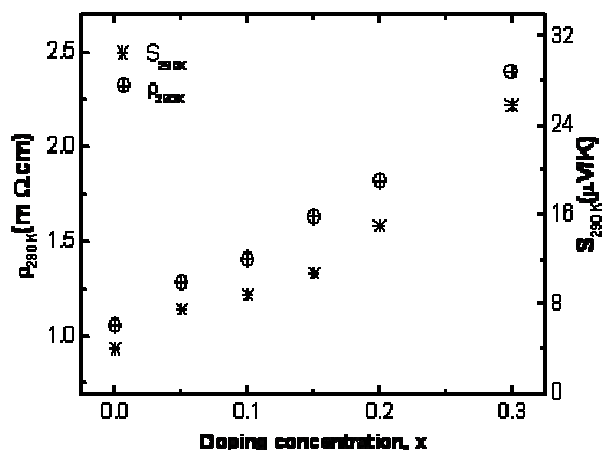
شکل ۳. وابستگی توان گرماالکتریسته و مقاومت ویژه الکتریکی در دمای اتاق به چگالی آلیش برای نمونه \text{Nd}_{1-x}\text{Pr}_x\text{Ba}_2\text{Cu}_2\text{O}_{7-\delta} .
