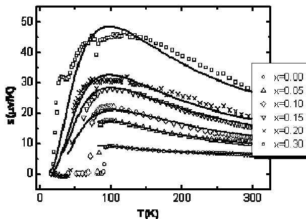
شکل ۲. وابستگی توان گرماالکتریسته به صورت تابعی از دما و تراکم آلیش برای نمونه \text{Nd}_{1-x}\text{Pr}_x\text{Ba}_2\text{Cu}_2\text{O}_{7-\delta} . خطوط توپر منحنی برازش داده‌های تجربی به مدل نوار باریک را نشان می‌دهد.
