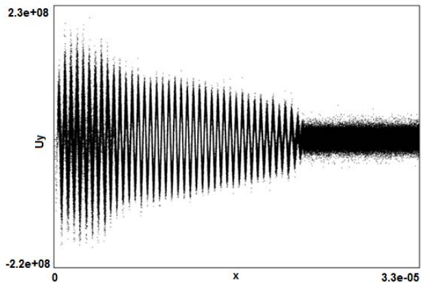
شکل ۱۳. فضای سرعت- مکان در جهت محور y در گام زمانی ۰.۱۱۲۳.
