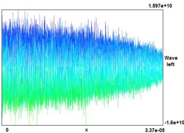
شکل ۱۲. امواج الکترومغناطیسی در جهت خلاف جهت محور x در گام زمانی ۲۵۴۷.
