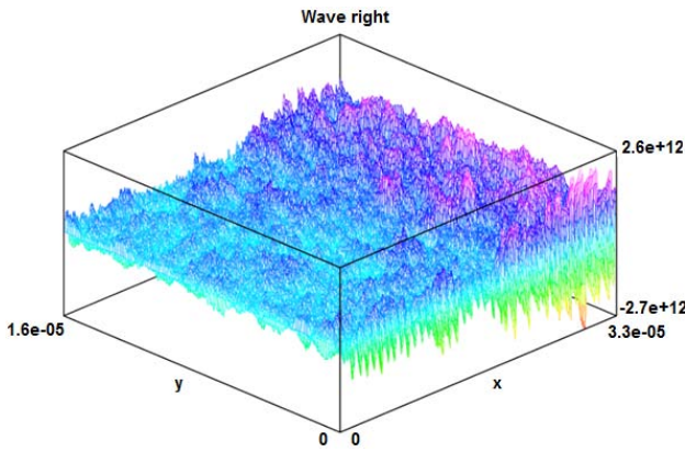
شکل ۱۰. امواج الکترومغناطیسی در جهت محور x در گام زمانی ۲۵۴۷.
