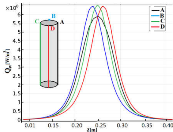
شکل ۱۱. (رنگی در نسخه الکترونیکی) نمودار گرمای حجمی قطعه کار برای پیچه تک حلقه‌ای در راستاهای A، B، C و D.
