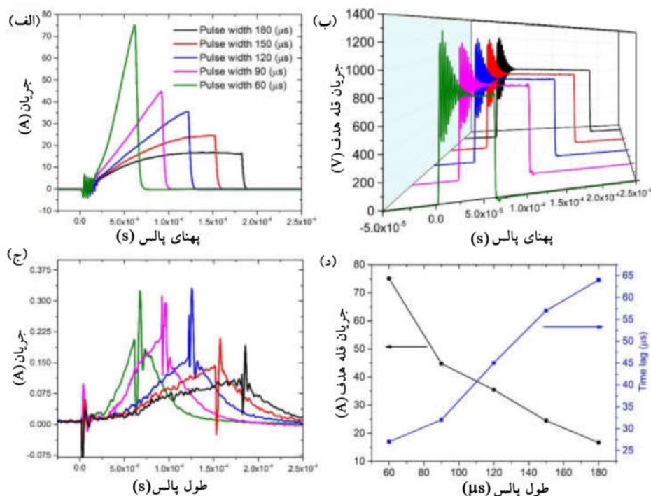
شکل ۲. (رنگی در نسخه الکترونیکی) (الف) منحنی‌های جریان و پتانسیل هدف و (ب) و منحنی جریان خالص زیرلایه. (ج) به صورت تابعی از پالس. (د) نمودار جریان پیشینه هدف و زمان تأخیر جریان خالص زیرلایه بر حسب پالس.
