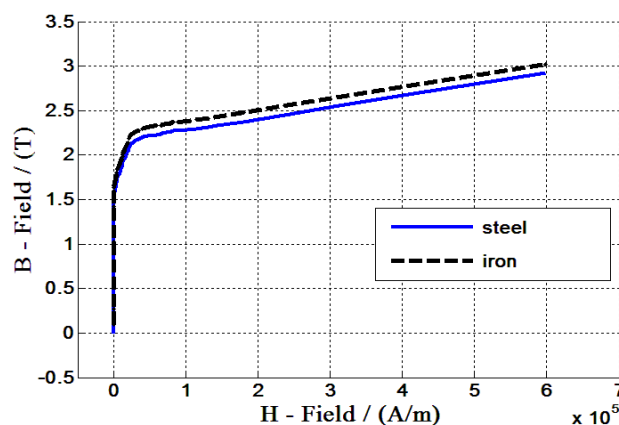
شکل ۵. تغییرات میدان مغناطیسی (B) بر حسب (H) برای آهن و استیل.
