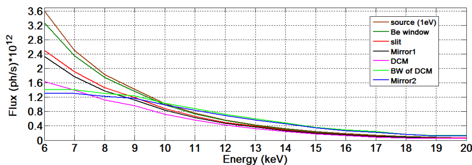
شکل ۳. مقدار شار ورودی به خط باریکه از چشمه و بعد از پنجره بریلیومی ( 200 \mu\text{m} )، بعد از شکاف ( 29 \times 2.1 \text{ cm}^2 ) آینه اول، تکفام کننده و آینه دوم (محاسبات با نرم افزار SPECTRA و Shadow انجام شده است).
