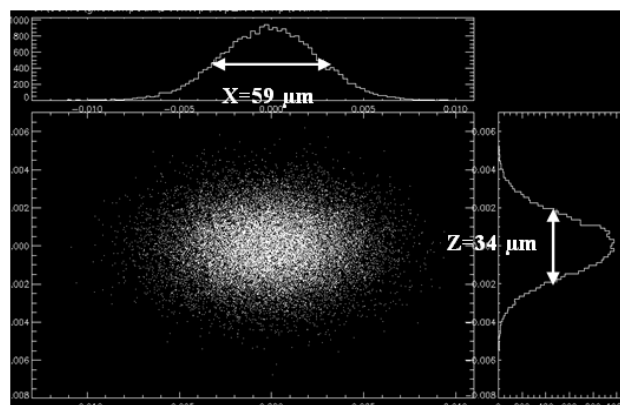
شکل ۲. اندازه و توزیع باریکه فوتونی در مکان نمونه با استفاده از Shadow (تعداد پرتوها ۲۵۰۰۰).
