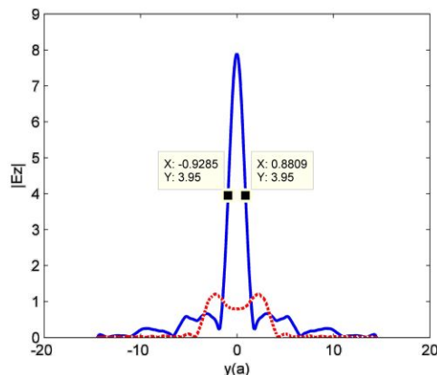
شکل ۴. (رنگی در نسخه الکترونیکی) اندازه میدان الکتریکی خروجی (منحنی پر رنگ) و ورودی (منحنی خط چین) بلور فوتونی دو بعدی متشکل از میله‌های سیلیکون در زمینه هوا با ثابت شبکه مدرج در بسامد \frac{wa}{2pc} = 0.39 برای مد TM.
