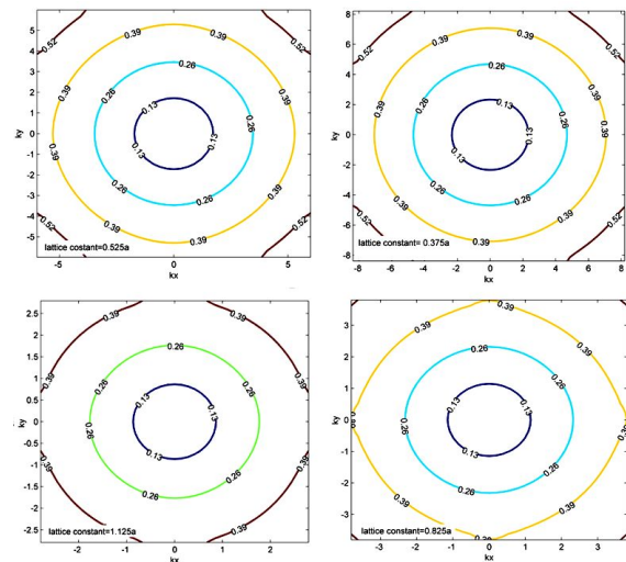
شکل ۴. (رنگی در نسخه الکترونیکی) منحنی‌های هم بسامد بلور فوتونی دو بعدی متشکل از میله‌های سیلیکون در زمینه هوا به ازای ثابت شبکه‌های برابر با 0.375a ، 0.525a ، 0.825a و 1.125a برای مد TM.
