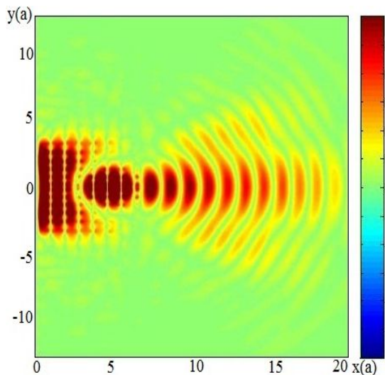
شکل ۳. (رنگی در نسخه الکترونیکی) توزیع فضایی میدان الکتریکی داخل بلور فوتونی با ثابت شبکه مدرج در بسامد \frac{wa}{2pc} = 0.39 برای مد TM.
