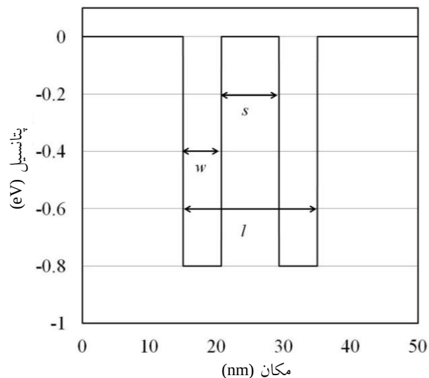
شکل ۱. چاه پتانسیل دوگانه ساده با نسبت فضای بین چاه به طول
