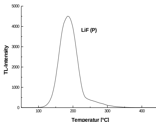
شکل ۶. منحنی گرمالیانی \text{LiF:P} بعد از پرتودهی با دز 100\text{ mGy} بتا.
