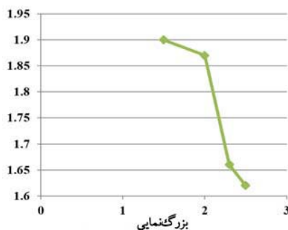
شکل ۱۴. (رنگی در نسخه الکترونیکی) کیفیت پرتوی محاسبه شده به صورت عددی برای لیزر در بزرگنمایی‌های ۱/۵، ۲، ۲/۳ و ۲/۵.
