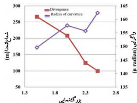
شکل ۱۳. (رنگی در نسخه الکترونیکی) شعاع انحنا و واگرایی باریکه محاسبه شده برای لیزر قرص در بزرگنمایی‌های ۱/۵، ۲، ۲/۳ و ۲/۵.
