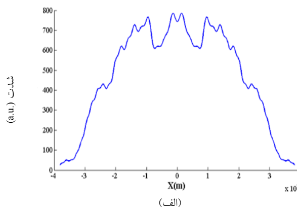
شکل ۱۷. (الف) مقطع شدت لیزر قرص نازک بدون لحاظ نمودن اثرات حرارتی، (ب) مقطع شدت لیزر قرص نازک با لحاظ نمودن اثرات حرارتی.
