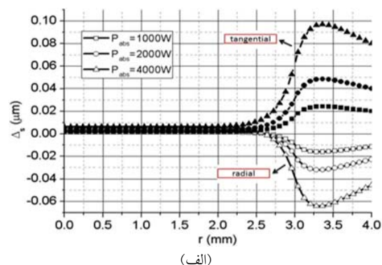
شکل ۹. (الف) نتایج OPD حاصل از کشش (اثر فوتوکشسان) برای دمش‌های مختلف ارائه شده در مرجع [۸]، (ب) نتیجه محاسبه OPD حاصل از کشش (اثر فوتوکشسان) برای دمش ۴۰۰۰ وات.
