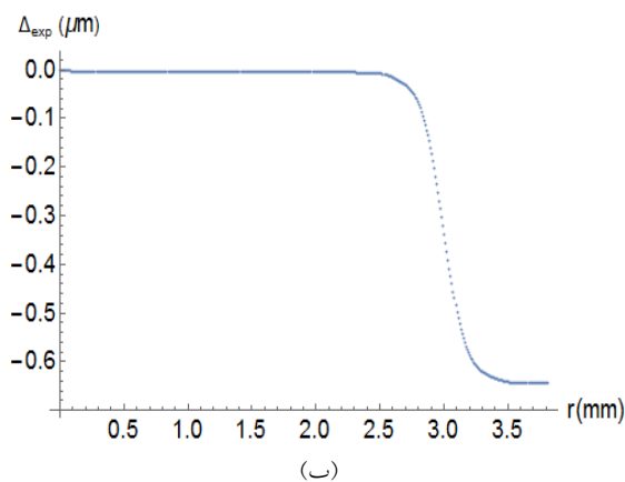
شکل ۸. (الف) نتایج OPD حاصل از انبساط حرارتی برای دمش‌های مختلف ارائه شده در مرجع [۸]، (ب) نتیجه محاسبه OPD حاصل از انبساط حرارتی برای دمش ۴۰۰۰ وات.
