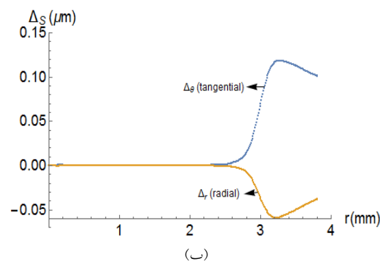
شکل ۹. (الف) نتایج OPD حاصل از کشش (اثر فوتوکشسان) برای دمش‌های مختلف ارائه شده در مرجع [۸]، (ب) نتیجه محاسبه OPD حاصل از کشش (اثر فوتوکشسان) برای دمش ۴۰۰۰ وات.
