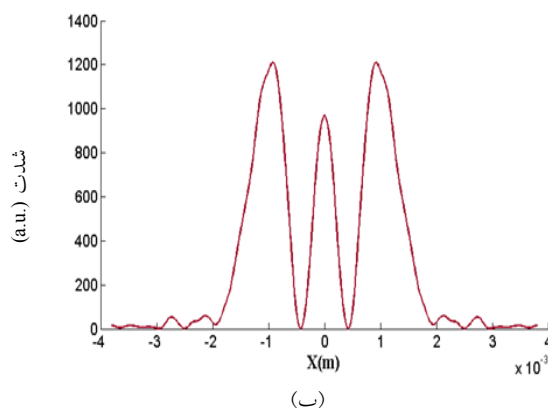
شکل ۱۷. (الف) مقطع شدت لیزر قرص نازک بدون لحاظ نمودن اثرات حرارتی، (ب) مقطع شدت لیزر قرص نازک با لحاظ نمودن اثرات حرارتی.
