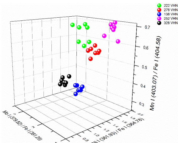
شکل ۷. (رنگی در نسخه الکترونیکی) تعدادی از متغیرهای تفکیک کننده آلیاژها با سختی متفاوت.
