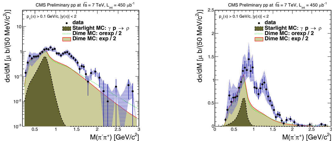
شکل ۳. (رنگی در نسخه الکترونیکی) سطح مقطع دیفرانسیلی یک جفت پایون از تابع جرم ناوردا، با مدل‌های پیش‌بینی شده داریم (به صورت خط مستقیم و نقطه-چین) مقایسه شده، که به مدل استرلایت (به صورت خط-چین) اضافه شده است.
