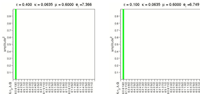
شکل ۳. (رنگی در نسخه الکترونیکی) احتمال حضور پروتون در توابع مجانبی در تشکیل یک ویژه حالت پرتونی با عدد پوسته‌ای N = 6 و \Omega = 13/2 در پارامترهای تغییر شکل کوچک و بزرگ.
