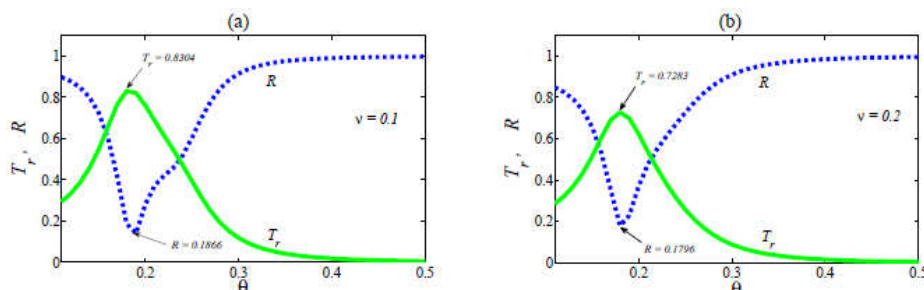
شکل ۲. (رنگی در نسخه الکترونیکی) نمودار ضرب عبور بر حسب زاویه برخورد برای دو مقدار بسامد برخورد متفاوت.
