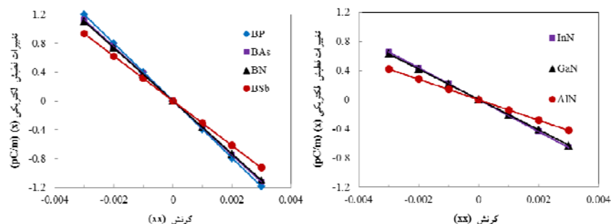
شکل ۶. (رنگی در نسخه الکترونیکی) نمودارهای تغییرات قطبش الکتریکی ایجاد شده در جهت x بر حسب کرنش‌های اعمالی در راستای xx
