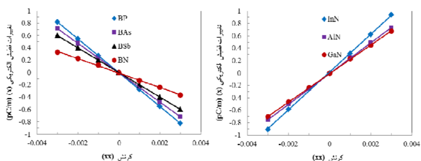
شکل ۷. (رنگی در نسخه الکترونیکی) نمودارهای تغییرات قطبش الکتریکی ایجاد شده در جهت x بر حسب کرنش‌های اعمالی در راستای xx
