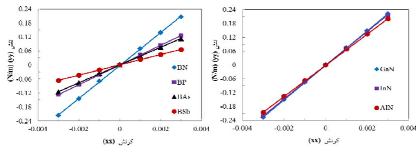
شکل ۵. (رنگی در نسخه الکترونیکی) نمودارهای تنش‌های صورت گرفته در جهت yy بر حسب کرنش‌های اعمالی در راستای xx برای حالت یون واهلش: شیب هر خط برابر ضریب کشسانی \tilde{C}_{12} یون واهلش ترکیب است.
