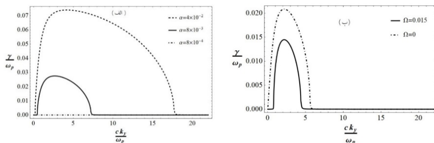
شکل ۵. نرخ رشد بی بعد شده \gamma / \omega_p ناپایداری رشته‌ای بر حسب عدد موج بی بعد شده K برای (الف) مقادیر مختلف نسبت چگالی الکترون‌های باریکه به الکترون‌های یون سپهر مغناطیده با \frac{\omega_c}{\omega_p} = 0.015 (ب) یون سپهر مغناطیده با \frac{\omega_c}{\omega_p} = 0.015 و غیرمغناطیده برای نسبت چگالی \alpha = 4 \times 10^{-3} . سایر کمیت‌ها \beta = 0.4 ، درجه یونش i = 10^{-3} و چگالی الکترون‌های یون سپهر n_e^0 = 10^6 \text{ cm}^{-3} انتخاب شده‌اند.
