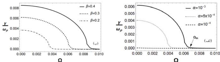
شکل ۳. نرخ رشد بی‌بعد شده ناپایداری رشته‌ای بر حسب بسامد سیکلوترونی الکترون (الف) برای سه مقدار مختلف \alpha ، 10^{-4} ، 10^{-3} ، 5 \times 10^{-4} ، 10^{-3} و سرعت ثابت \beta = 0.3 ، (ب) برای مقادیر مختلف \beta ، 0.2 ، 0.3 و 0.4 در چگالی ثابت \alpha = 10^{-3} . K = 1 و سایر کمیت‌ها همانند شکل ۱ (ب) انتخاب شده‌اند.
