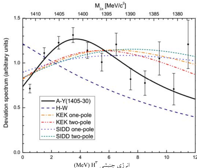
شکل ۶. (رنگی در نسخه الکترونیکی) طیف انحراف توزیع انرژی جنبشی ترایتون آزاد شده (جرم ناوردای (\Sigma\pi)^\circ ) در برهم‌کنش (K^- \rightarrow \bar{K}^0 \pi^+ \pi^-) برای پتانسیل‌های پدیده‌شناختی A-Y، تک‌قطبی و دوقطبی SIDD [۳۴] و KEK [۳۵]، و پتانسیل کایرال هیدو-وایز [۱۸] با قطب‌های انرژی متفاوت \Lambda(1405) .
