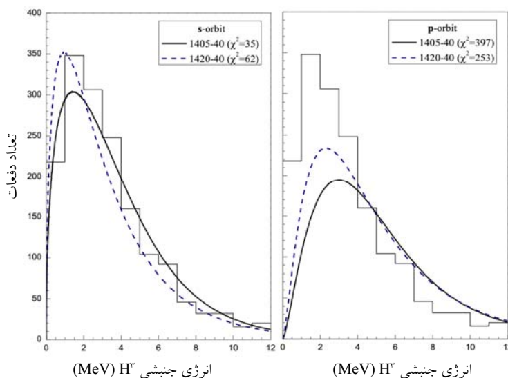
شکل ۱. برازش طیف‌های انرژی جنبشی ترایتون ناشی از جذب تشدید K^- در {}^4\text{He} ، بر طیف تجربی (نمودار پله‌ای). طیف‌های نظری ناشی از جذب از اوربیتال‌های اتمی s (سمت چپ) و p (سمت راست)، به ازای M_{\Lambda^*} = 1405 (خطوط توپر) و M_{\Lambda^*} = 1420 (خطوط خط‌چین) با پهنای ۴۰ MeV محاسبه شده‌اند. مقدار \chi^2 برای هر مورد در شکل نشان داده شده است.
