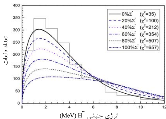
شکل ۲. برآزش طیف‌های انرژی جنبشی، تراکتون بر داده‌های تجربی (نمودار یله‌ای)، به ازای جمعیت‌های مختلف تشدید (۱۳۸۵) \Sigma^* .
