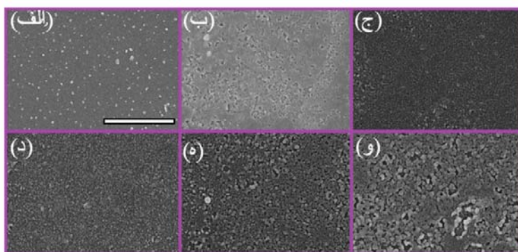
شکل ۳. (رنگی در نسخه الکترونیکی) تصاویر SEM از لایه \text{ZnS}(n) رسوب داده شده بر روی زیرلایه \text{PbS}(3) ، با تعداد چرخه پوشش‌دهی (الف) n=0 ، (ب) n=2 ، (ج) n=4 ، (د) n=6 ، (ه) n=8 و (و) n=10 . نوار مقیاس: ۱ میکرومتر.
