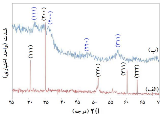
شکل ۲. (رنگی در نسخه الکترونیکی) الگوی پراش پرتوی ایکس؛ (الف) \text{PbS}(3) و (ب) \text{ZnS}(6) .
