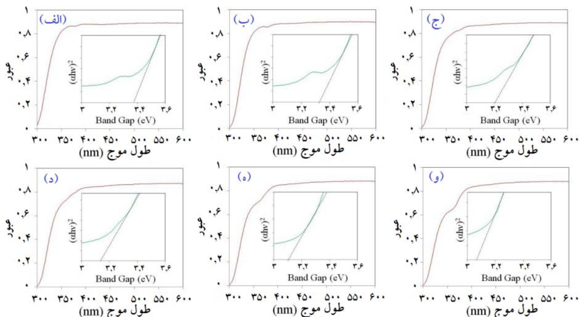
شکل ۵. (رنگی در نسخه الکترونیکی) عبور نور از لایه‌های \text{PbS}(3)/\text{ZnS}(n) با n=0 (الف) (ب) ۲، (ج) ۴، (د) ۶، (ه) ۸ و (و) ۱۰، که بر روی بسترهای شیشه‌ای لایه‌نشانی شده‌اند. ضمیمه‌های هر شکل، نمودار (\alpha h\nu)^2 بر حسب h\nu را نشان می‌دهد.
