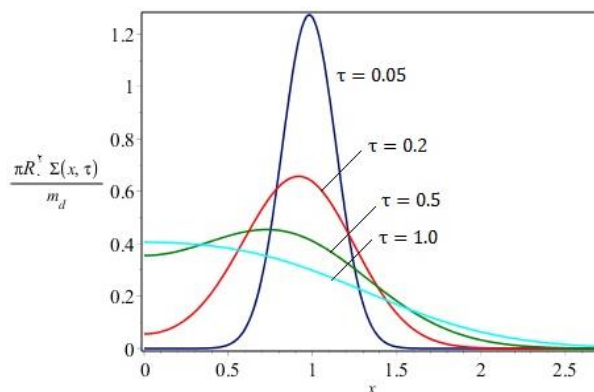
شکل ۴. (رنگی در نسخه الکترونیکی) سیال حلقه‌ای دارای جرم اولیه m_d و شعاع اولیه R_* است. چگالی سطحی \Sigma تابعی از مکان و زمان بدون بعد است. در این شکل پخش شدن حلقه اولیه در اثر وشکسانی به وضوح دیده می‌شود.
