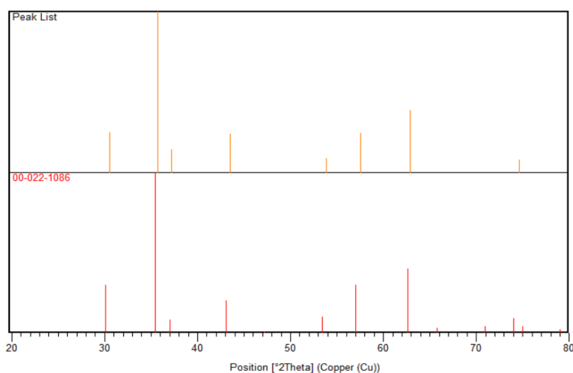
شکل ۳. (رنگی در نسخه الکترونیکی) تطبیق زوایای پراش الگوی پراش پرتو ایکس نمونه 400^\circ\text{C} با کارت استاندارد با استفاده از نرم‌افزار X'pert.
