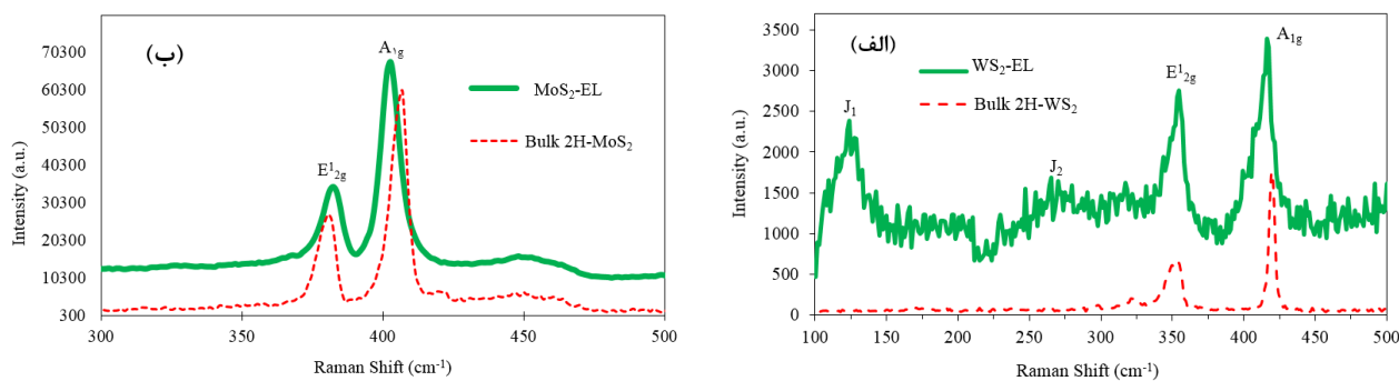
شکل ۶. (رنگی در نسخه الکترونیکی) طیف رامان نانوصفحات سنتز شده: (الف) نمونه WS_2 -EL و (ب) نمونه MoS_2 -EL. طیف رامان استاندارد توده WS_2 و MoS_2 نیز در هر نمودار برای مقایسه، رسم شده است.
