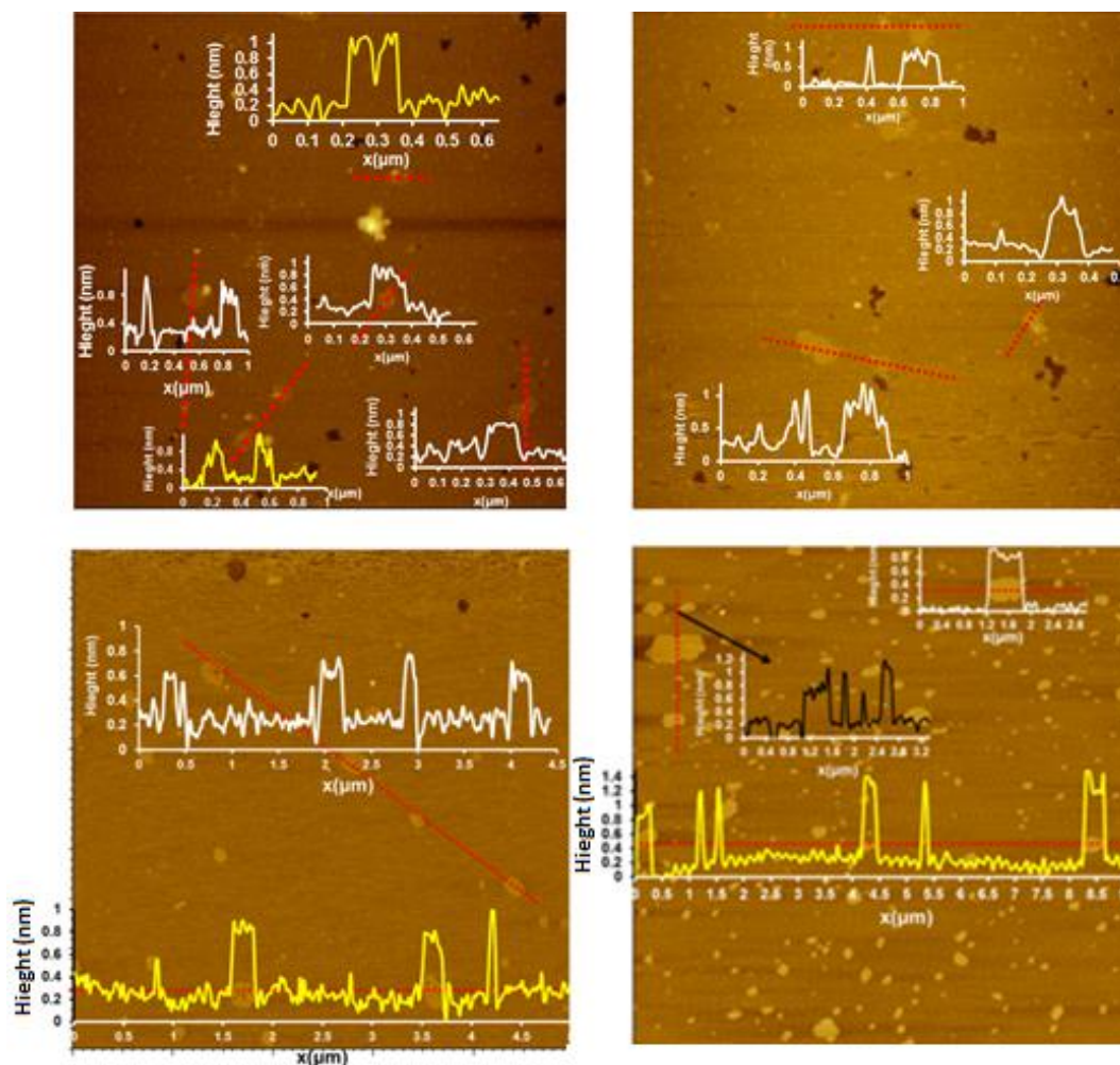
شکل ۴. (رنگی در نسخه الکترونیکی) تصاویر دوبعدی AFM به همراه پروفایل‌های مربوطه (نشان دهنده ضخامت هر صفحه)، به دست آمده از نانوصفحات تک لایه \text{MoS}_2 (دو تصویر بالایی)، و \text{WS}_2 (دو تصویر پایینی).
