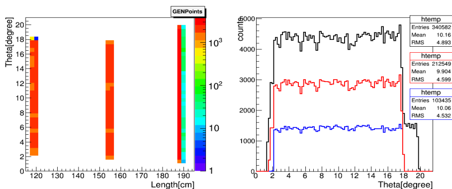
شکل ۱. (رنگی در نسخه الکترونیکی) شکل سمت چپ توزیع زاویه‌ای ناحیه فعال هر سه ایستگاه آشکارساز ردیاب تکثیر کننده الکترون گازی (نمودار زاویه قطبی تنا بر حسب مکان Z لایه‌های حساس هر ایستگاه) و شکل سمت راست نمودار شمارش ذرات بر حسب زاویه قطبی تنا به ترتیب برای ایستگاه اول به تنهایی (آبی)، برای ایستگاه اول و دوم با هم (قرمز) و برای هر سه ایستگاه با هم (سیاه) را نشان می‌دهند.
