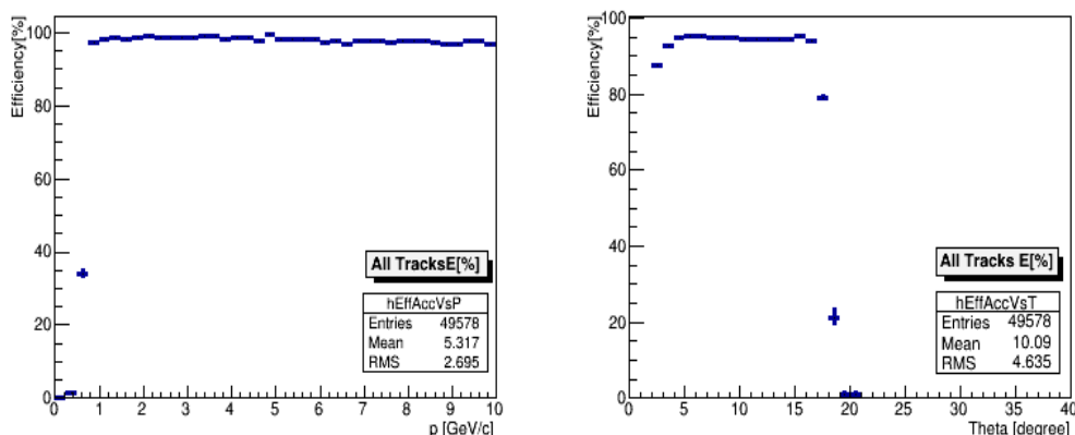
شکل ۳. (رنگی در نسخه الکترونیکی) سمت راست: نمودار توزیع زاویه‌ای، سمت چپ: نمودار توزیع تکانه برای بازده ردیابی GEM.
