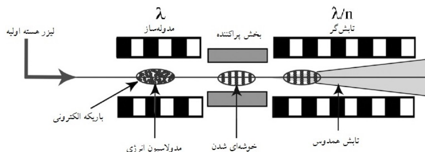
شکل ۱. ساختار کلی کلاسترون نوری.
