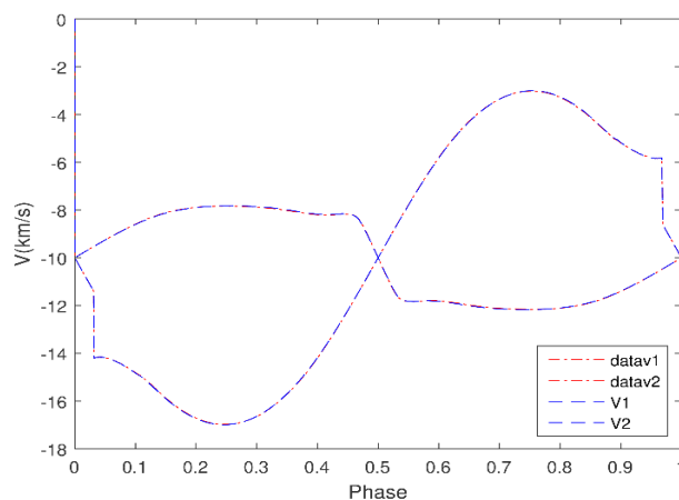
شکل ۵. (رنگی در نسخه الکترونیکی) منحنی‌های سرعت شعاعی دستگاه نمونه بر حسب فاز رسم شده‌اند \text{datav}_1 و \text{datav}_2 منحنی‌های سرعت شعاعی دستگاه نمونه برای کمیت‌های روشنایی سطحی دقیق محاسبه شده هستند، و V_1 و V_2 منحنی‌های سرعت شعاعی با ضرایب روشنایی سطحی به دست آمده از طیف سنجی هستند.
