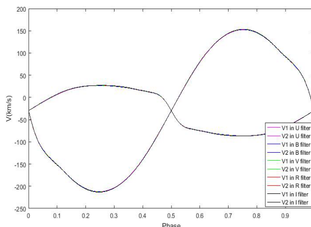
شکل ۷. منحنی‌های سرعت شعاعی دوتایی U Peg که در صافی‌های مختلف I, R, V, B, U رسم شده است.
