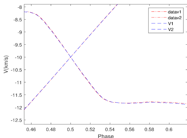
شکل ۶. (رنگی در نسخه الکترونیکی) منحنی‌های سرعت شعاعی دستگاه نمونه که درشت‌نمایی شده بر حسب فاز در اطراف فاز ۰٫۵ رسم شده‌اند. \text{datav}_1 و \text{datav}_2 منحنی‌های سرعت شعاعی دستگاه نمونه برای ضرایب روشنایی سطحی دقیق محاسبه شده هستند، و V_1 و V_2 منحنی‌های سرعت شعاعی با ضرایب روشنایی سطحی به دست آمده از طیف سنجی هستند.
