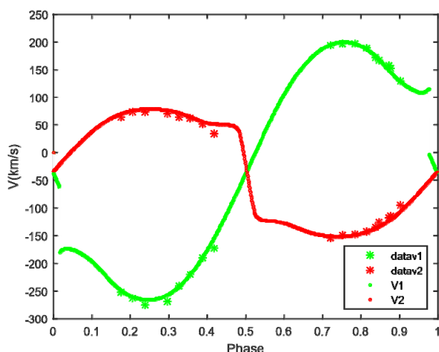
شکل ۱۱. (رنگی در نسخه الکترونیکی) منحنی‌های مشاهداتی و محاسباتی سرعت‌های شعاعی ستارگان اولیه و ثانویه بر حسب فاز دستگاه دوتایی BD+422782. داده‌های مشاهداتی از [۱۱] است.
