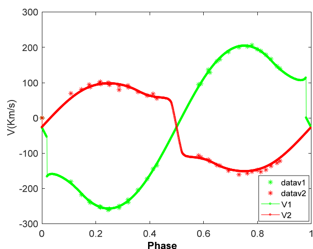
شکل ۱۰. (رنگی در نسخه الکترونیکی) منحنی‌های مشاهداتی و محاسباتی سرعت‌های شعاعی ستارگان اولیه و ثانویه بر حسب فاز دستگاه دوتایی AB And. داده‌های مشاهداتی از [۱۰] است.
