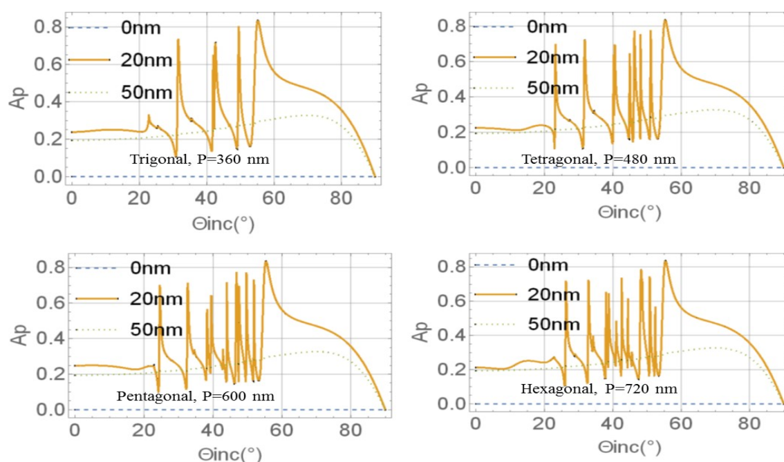
شکل ۳. (رنگی در نسخه الکترونیکی) نمودارهای جذب اپتیکی قطبش P محاسبه شده برای ۲ پریود گام ساختاری برای لایه‌های نازک کایرال ۳، ۴، ۵ و شش‌گوشی به ازای ضخامت‌های متفاوت لایه نازک فلزی. در محاسبات t_{STF} = 2P و \chi_v = 30^\circ در نظر گرفته شده است.
