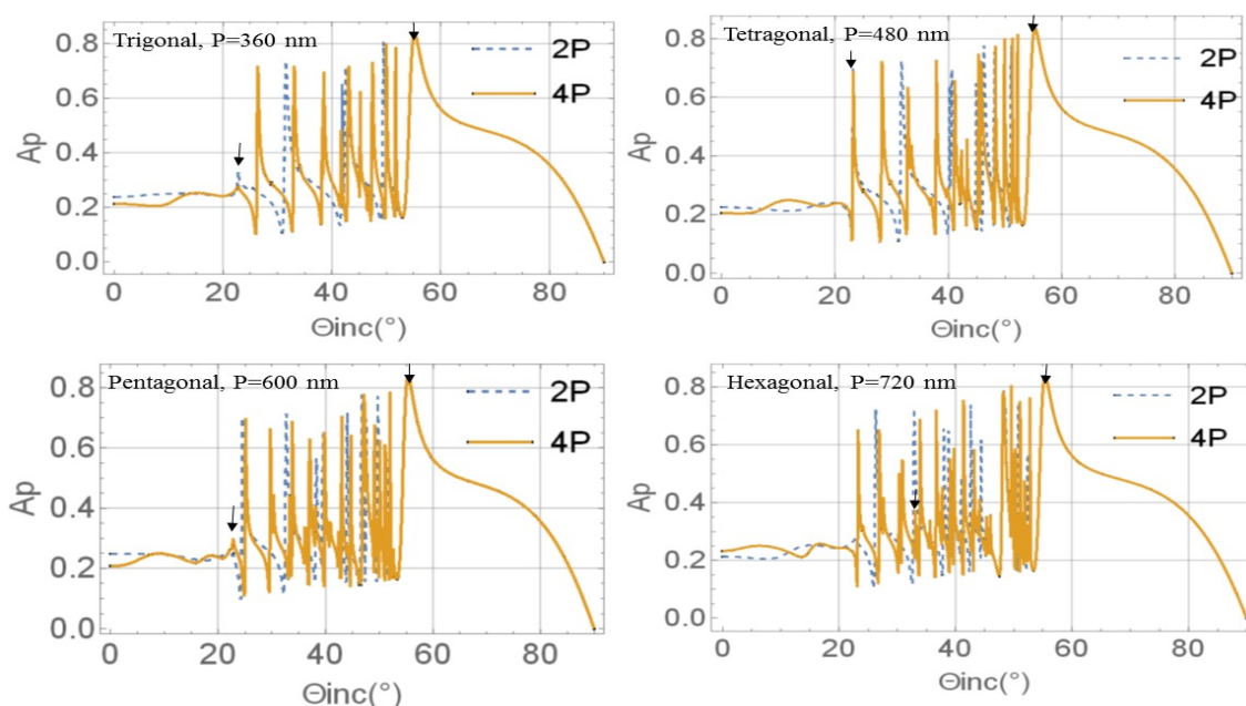
شکل ۲. (رنگی در نسخه الکترونیکی) نمودارهای جذب اپتیکی قطبش P محاسبه شده برای ۲ و ۴ پریود گام ساختاری برای لایه‌های نازک کایرال ۳، ۴، ۵ و شش‌گوشی. در محاسبات t_{Met} = 20 \text{ nm} و \chi_v = 30^\circ در نظر گرفته شده است.
