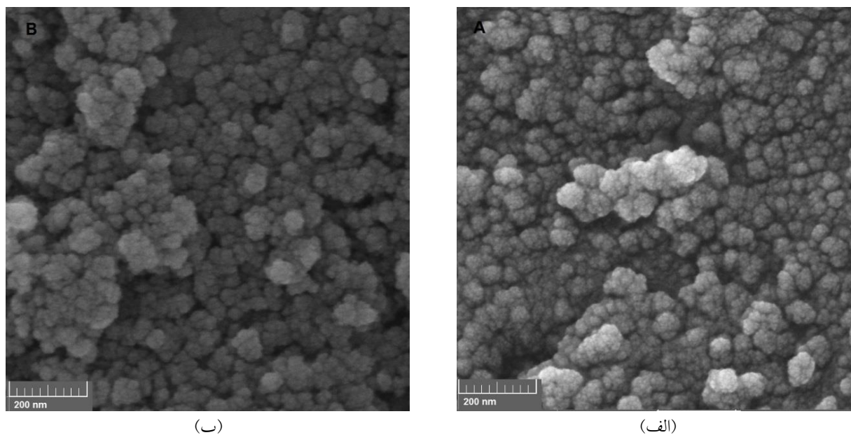
شکل ۲. تصاویر FESEM در مقیاس ۲۰۰ nm، (الف) نمونه آب‌گریز و (ب) نمونه آب‌دوست.
