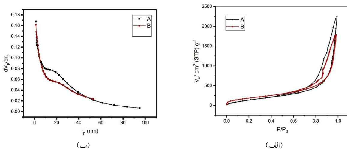
شکل ۵. (الف) نمودارهای جذب و واجذب گاز نیتروژن و (ب) نمودارهای توزیع اندازه حفره‌های دو نمونه A و B.
