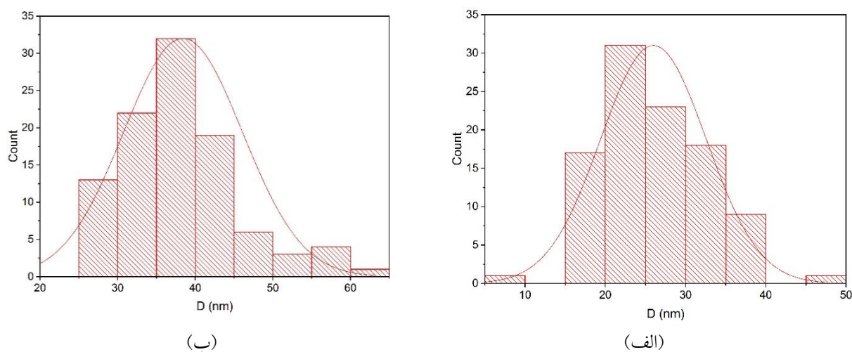
شکل ۳. نمودار توزیع اندازه ذرات با استفاده از دیجیمایزر، (الف) نمونه آب‌گریز و (ب) نمونه آب‌دوست.
