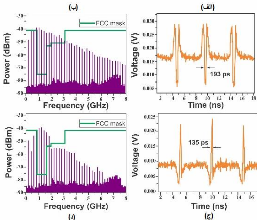
شکل ۶. تولید پالس‌های دوتایی باند فرابنفش. (الف) پالس‌های دوتایی در طول موج تشدید که برابر ۱۵۴۸/۹۳ نانومتر است، (ب) طیف الکتریکی آن، (ج) پالس‌های دوتایی در طول موج تشدید که برابر ۱۵۵۳/۷۴ نانومتر است و (د) طیف الکتریکی آن.
