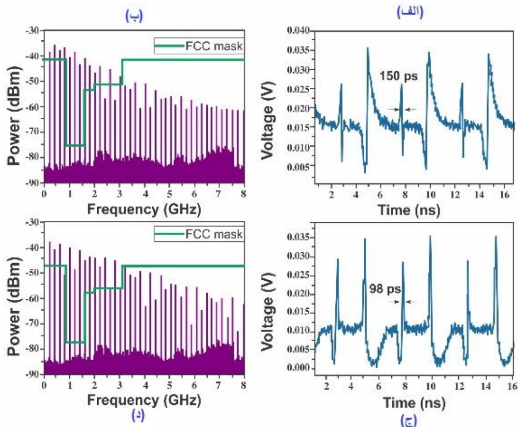
شکل ۵. تولید پالس‌های تک‌چرخه‌ای باند فراپهن. (الف) پالس‌های تک‌چرخه‌ای در طول موج تشدید که برابر 1548/93 نانومتر است، (ب) طیف الکتریکی آن، (ج) پالس‌های تک‌چرخه‌ای در طول موج تشدید که برابر 1553/74 نانومتر است و (د) طیف الکتریکی آن.
