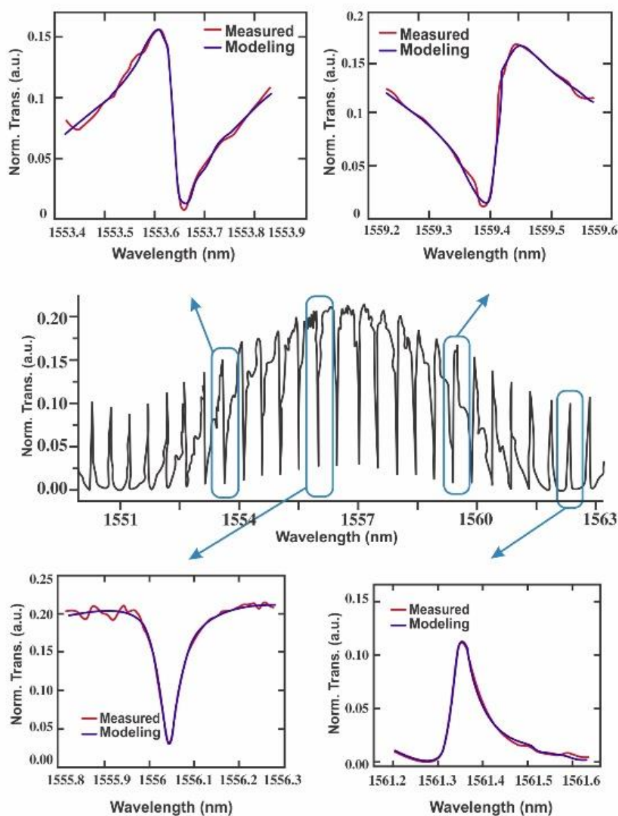
شکل ۳. عبور اندازه‌گیری شده طیف تداخل سنج ماخ‌زندر با یک تشدیدگر حلقه‌ای کوچک در یک چرخه تکامل تشدید. الحاقیات، طیف تشدید بزرگنمایی شده در طول موج‌های مختلف را نشان می‌دهند. طیف مدل‌سازی شده هم نشان داده شده است.
