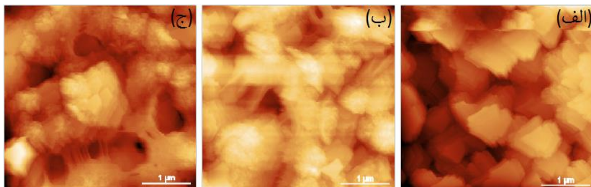
شکل ۴. تصاویر میکروسکوپ نیروی اتمی از غشاهای (الف) PVDF، (ب) PGO-۰/۳٪ و (ج) PGO-۰/۵٪.
