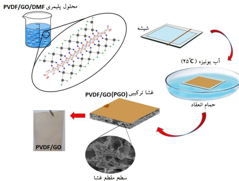
شکل ۱. مراحل ساخت غشاهای PVDF و PGO به روش تبدیل فاز- غوطه‌وری در آب.
