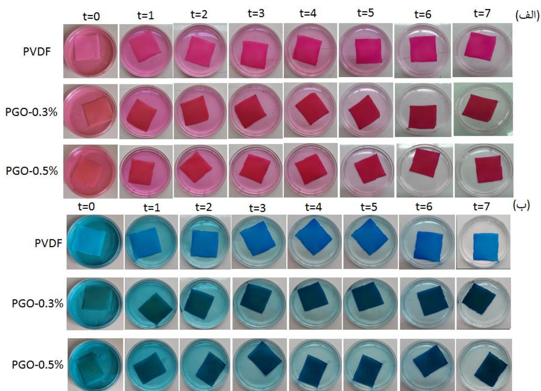
شکل ۹. تصاویر اپتیکی از فرایند جذب رنگدانه‌ها بر روی غشاهای PVDF، PGO-۰/۳٪ و PGO-۰/۵٪ در طول ۷ ساعت، (الف) رنگدانه RB و (ب) رنگدانه MB.
