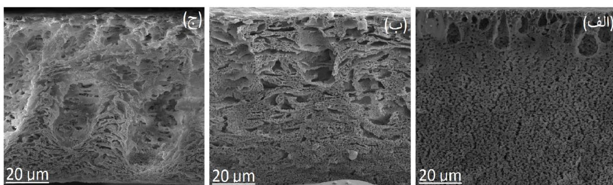
شکل ۵. تصاویر میکروسکوپ الکترونی روبش از غشاهای (الف) PVDF، (ب) PGO-۰/۳٪ و (ج) PGO-۰/۵٪.
