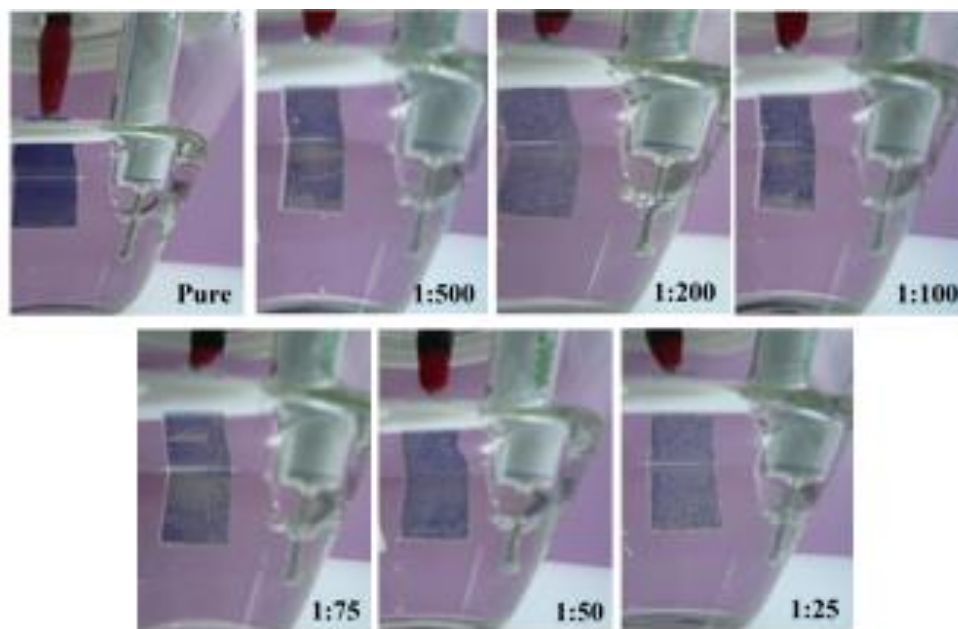
شکل ۱۰. تصاویر موقعیت رنگی نمونه‌های WO_3 -Pd با نسبت‌های مولی مختلف برای Pd:W (تصاویر مربوط به موقعیت رنگی نمونه‌ها در پتانسیل اعمالی ۱/۲ V- است).
