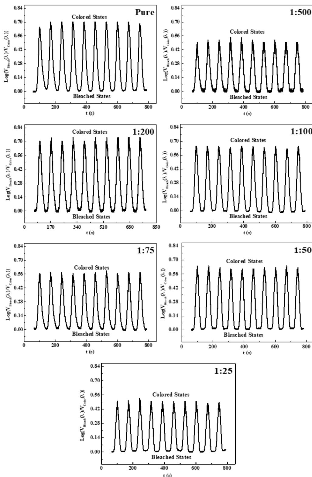
شکل ۷. تغییرات چگالی اپتیکی نمونه‌های \text{WO}_3 خالص و \text{WO}_3/\text{Pd} طی فرایند رنگی/شفاف شدن الکتروکرومیک در بازه پتانسیل اعمالی [+0.6 \text{ V} \leftarrow -1.2 \text{ V}] و برای لیزر (He-Ne) با طول موج 632.8 \text{ nm} .
