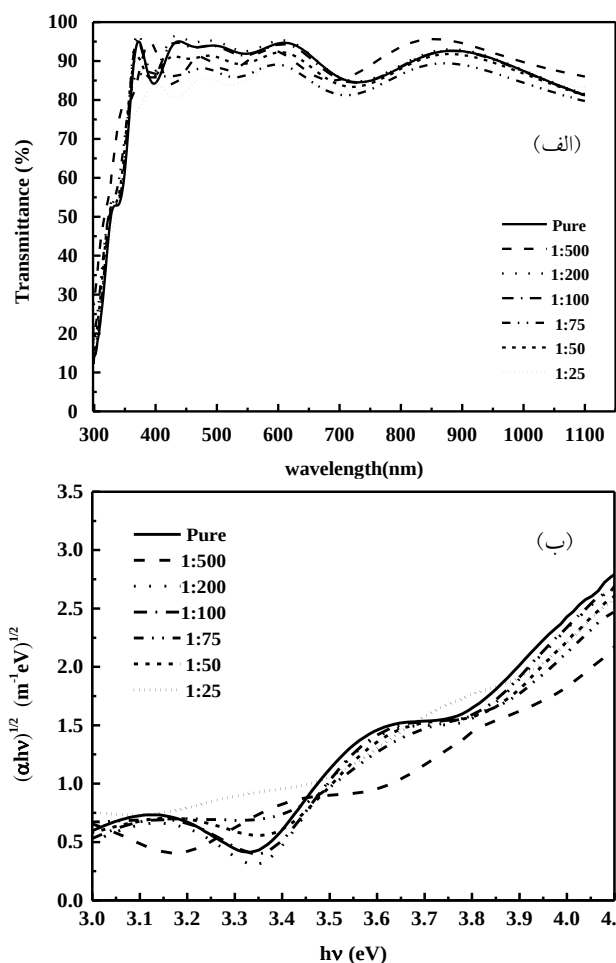
شکل ۴. (الف) طیف عبور اپتیکی و (ب) منحنی‌های (\alpha h\nu)^{1/2} برحسب h\nu برای حالت شفاف لایه‌های نازک WO_3 خالص و WO_3 -Pd با نسبت‌های مولی مختلف برای Pd:W.
