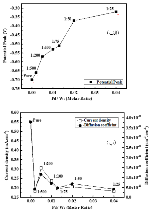
شکل ۶. (الف) موقعیت پتانسیل مربوط به قله جریان کاتدی در نمودار ولتاموگرام و (ب) چگالی جریان کاتدی و ضریب نفوذ شیمیایی برحسب نسبت‌های مولی مختلف Pd نمونه‌های WO 3 و WO 3 -Pd.
