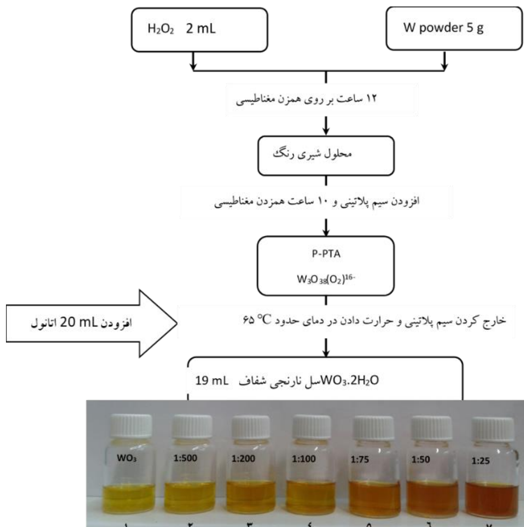
شکل ۱. سل تنگستیک اسید خالص ( \text{WO}_3 ) و سل تنگستیک اسید آرایش یافته با پالادیم ( \text{WO}_3\text{-Pd} ) در نسبت‌های مولی مختلف ۱:۵۰۰، ۱:۲۰۰، ۱:۱۰۰، ۱:۷۵، ۱:۵۰ و ۱:۲۵ برای \text{Pd:W} ، به ترتیب از چپ به راست.
