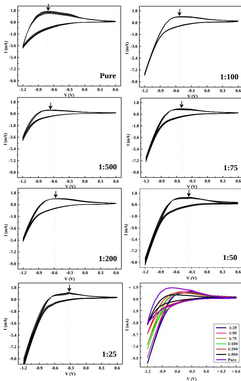
شکل ۵. ده چرخه اول منحنی‌های ولتامتری چرخه‌ای نمونه‌های \text{WO}_3 خالص و \text{WO}_3\text{-Pd} با غلظت‌های مولی مختلف برای \text{Pd:W} ، با سرعت روبش 50 \text{ mV.s}^{-1} در محلول 5 \text{ mM} \text{H}_2\text{PO}_4 / ۰٫۵ مولار. مقایسه مشخصه‌های چرخه اول منحنی‌های ولتاموگرام نیز نشان داده شده است.
