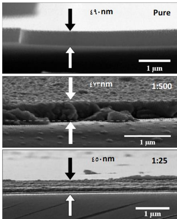
شکل ۳. تصاویر SEM از مقاطع عرضی لایه‌های نازک \text{WO}_3 خالص و \text{WO}_3 -Pd با غلظت‌های مولی ۱:۵۰۰ و ۱:۲۵. دقت اندازه‌گیری ضخامت (\pm 8 \text{ nm}) .
