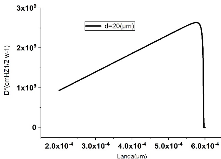
شکل ۵. نمودار آشکارسازی نمونه بهینه شده در دمای ۳۰۰ کلوین.
