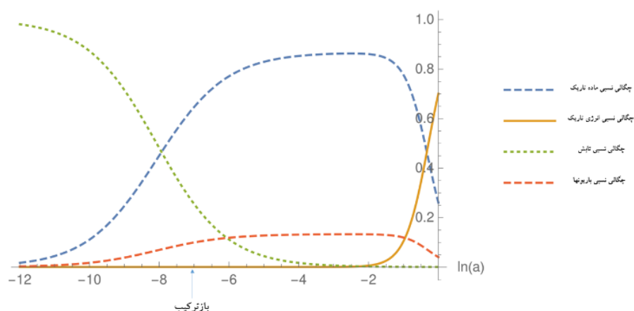
شکل ۲. چگالی نسبی مؤلفه‌های گوناگون بر حسب لگاریتم طبیعی عامل مقیاس برای حالت \xi = 0 یا همان مدل استاندارد \Lambda CDM.
