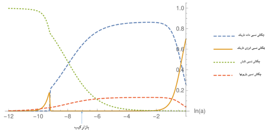
شکل ۱. تحول چگالی نسبی مؤلفه‌های گوناگون بر حسب لگاریتم طبیعی عامل مقیاس برای حالت \xi = e^{-\tau} . همان طور که روشن است در زمان قبل از بازترکیب، انرژی تاریک چگالی نسبی قابل اعتنا نباشد و فاز انرژی تاریک اولیه پدیدار می‌شود. با افزایش آهنگ برهمکنش، زمان بروز این فاز به زمان حال نزدیک‌تر می‌شود.
